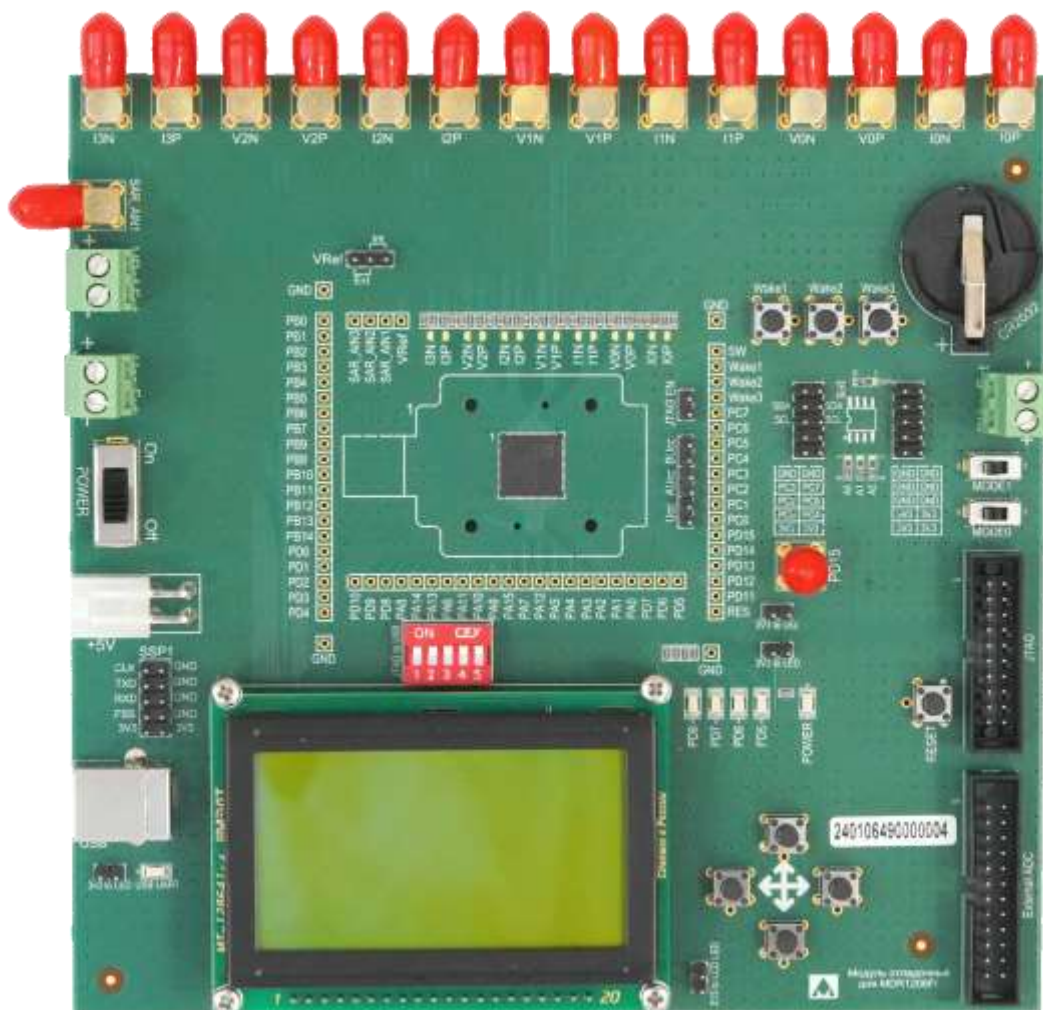
Рисунок 2 – Вид изделия без упаковки со стороны микросхемы MDR1206FI *
